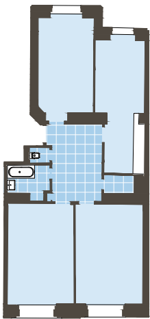
Stávající dispozice
