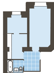
Stávající dispozice
